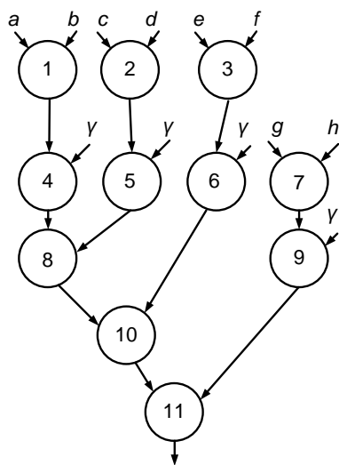
Рис. 4. Граф задачи
