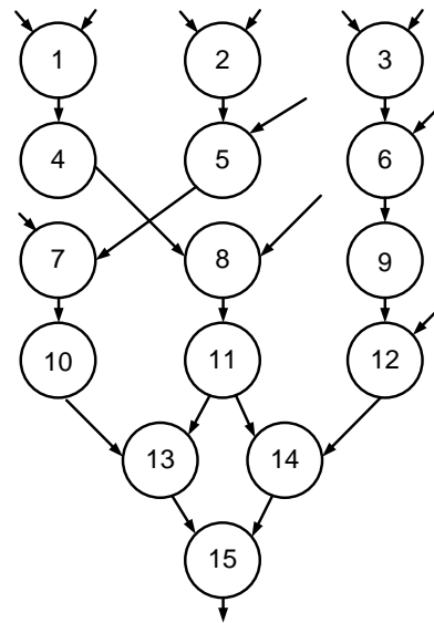
Рис. 1. Граф задачи
